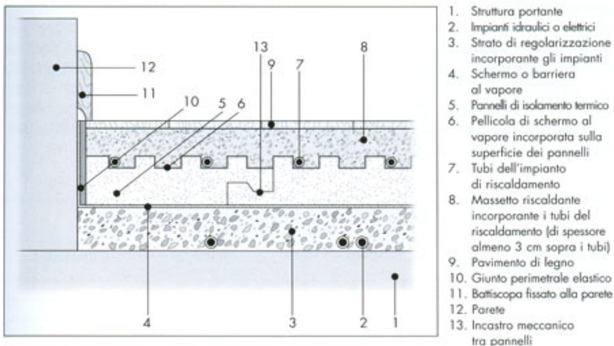
Schema tipico di un pavimento riscaldato
